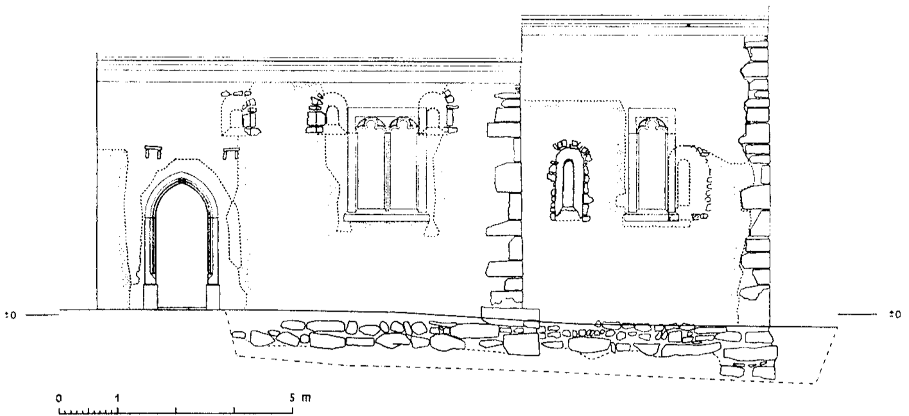
8 Ansicht der Südwand außen.
