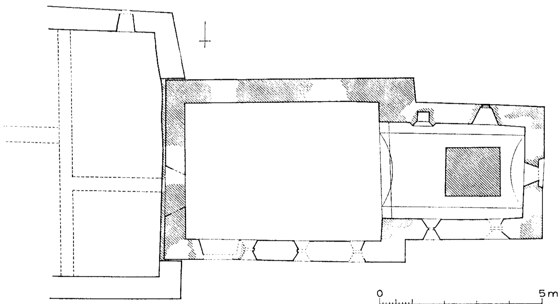
6 Rekonstruktionsgrundriß Periode IV.
