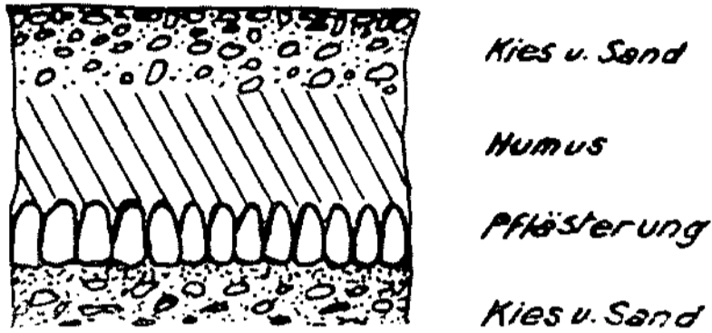
Fig. 6. Querschnitt durch das vermutlich römische Straßenpflaster bei Weinfelden. Gezeichnet von J. Thalman, Nachführungsgeometer.
